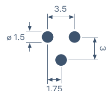
Maßstab 2:1 Scale 2:1
