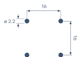
Maßstab 1:1 Scale 1:1
