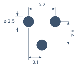
Maßstab 2:1 Scale 2:1
