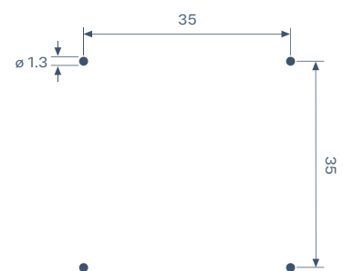
Maßstab 1:1 Scale 1:1
