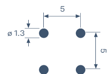
Maßstab 2:1 Scale 2:1
