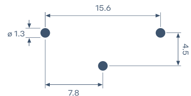
Maßstab 2:1 Scale 2:1
